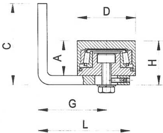
BOTTOM HINGE
