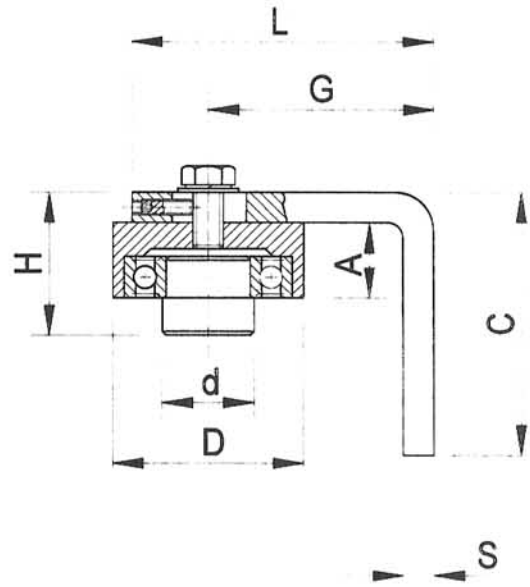
TOP HINGE
